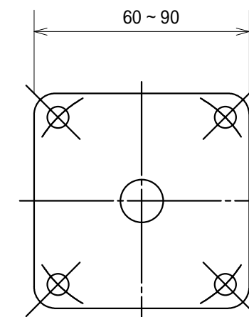
フランジ形状一例
